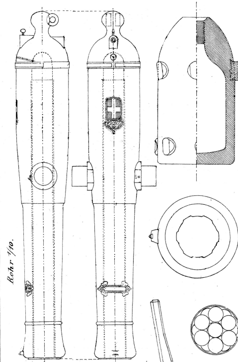
Italienische 6 28 re kanone.
