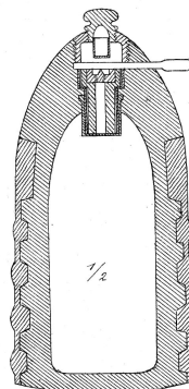
Projekt nebst Zünder.
