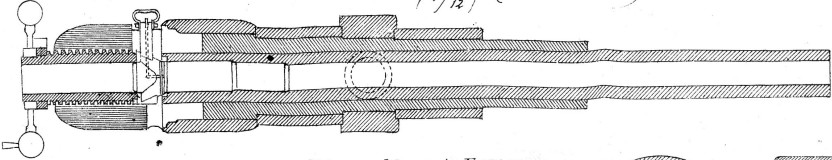
Filzvoranschlag mit Fettkapsel
