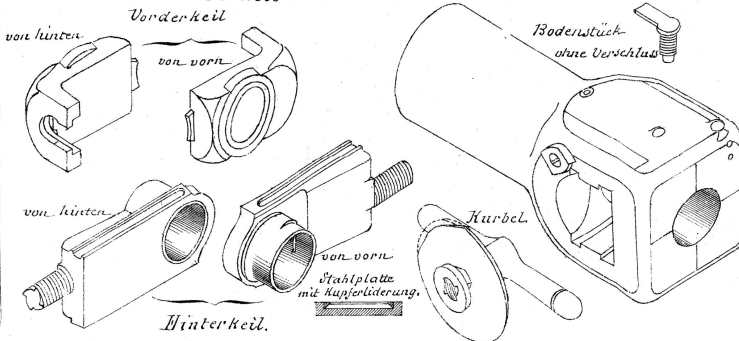
Englisches gez. 12 8ges Rohr. (Armstrong)
