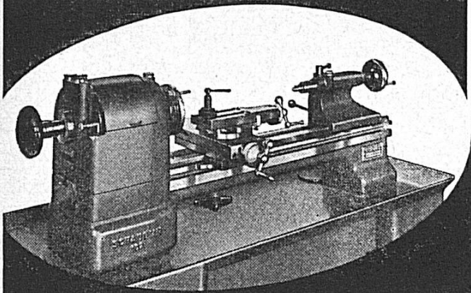
TOUR OUTILLEUR
