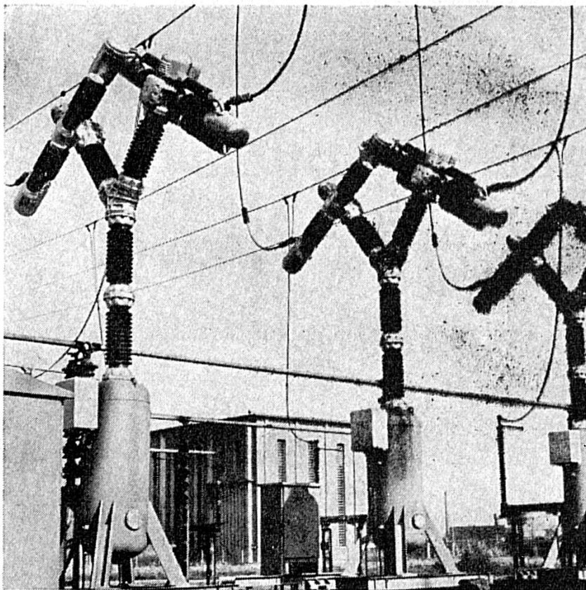
Disjoncteurs pneumatiques BBC, type DLF pour montage à l'extérieur
