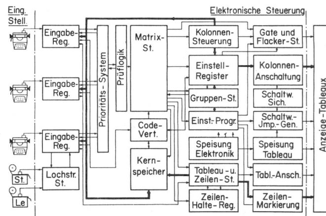
Fig. 9 Vereinfachtes Blockschaftbild der Eingabe- und Steuerausüstung einer Flugmeldeanlage
