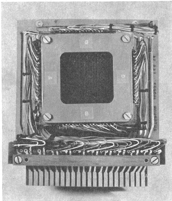
Fig. 8 Ferritkernspeicher mit je 1024 Ringkernen in 5 Ebenen zur Speicherung von z. B. 1024 Wörtern von je 32 Buchstaben
