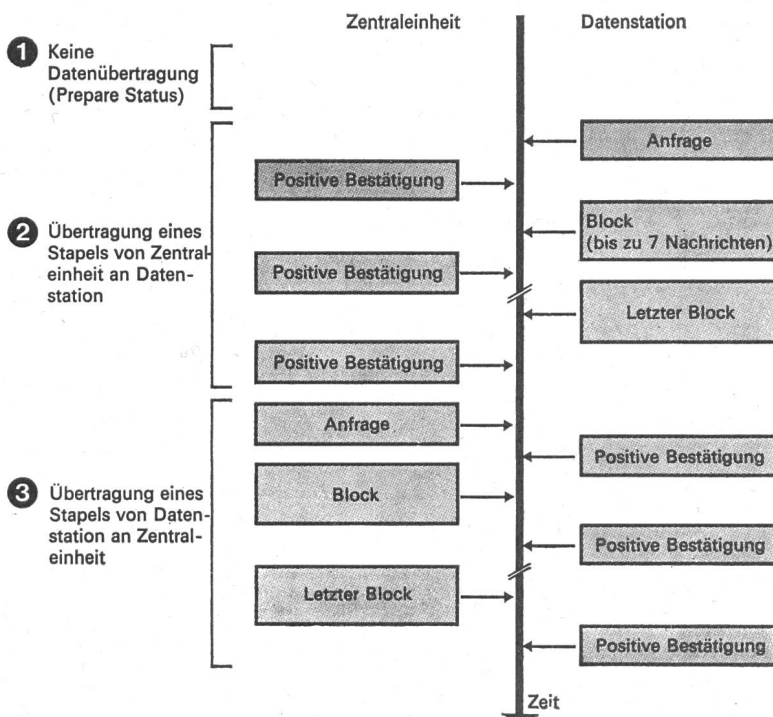
Fig. 7 Beispiel eines Ablauf-(polling)systems Sowohl die Zentraleinheit als auch die Datenstationen können sich gegenseitig befragen und entsprechende Antworten geben. Eine Aufrufoutine verhindert die falsche Zuordnung von Meldungen und Stationen; die Übertragung selbst kann blockweise vor sich gehen, damit die zur Korrektur von eventuell auftretenden Übertragungsfehlern notwendige Speicherkapazität klein gehalten werden kann
