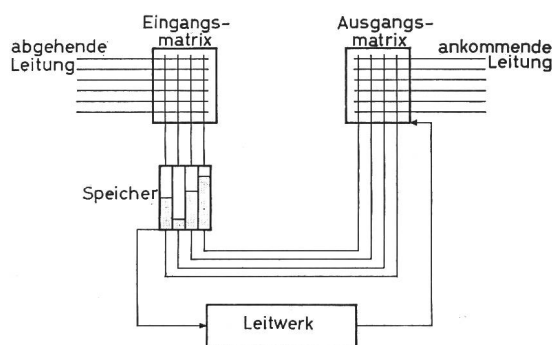
Fig. 12 Prinzipschema einer adressengesteuerten Speichervermittlung Eine ankommende Meldung (Telegramm) wird einer freien Speicherzelle zugeführt und von dort bei Freiwerden der entsprechenden Ausgangsleitung abgerufen. Das Leitwerk besorgt die Haushaltfunktionen (Prioritäten, queues, Leitwege und Abrechnung)
