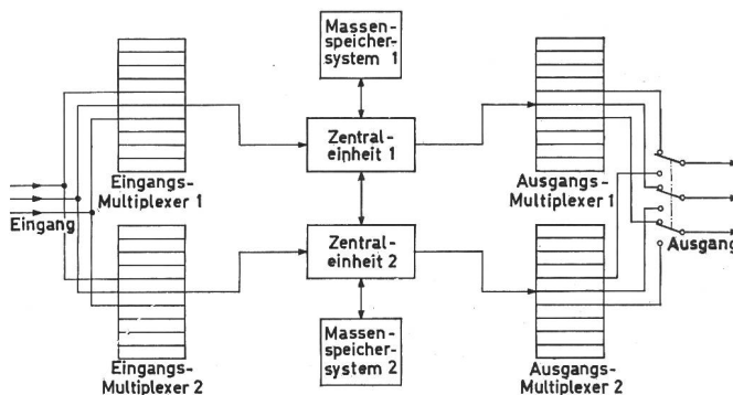
Fig. 13 Dualsystem einer Speichervermittlung Die beiden eingangsseitig parallel geschalteten Anlagen müssen ablaufmässig miteinander gekoppelt werden, damit die ausgangsseitig erfolgende Umschaltung von der Betriebs- auf die Reserveanlage ohne Informationsverlust erfolgen kann
