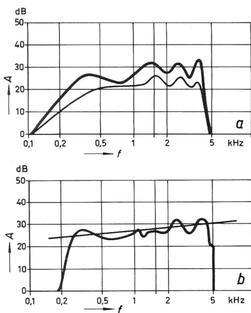
Fig. 3 Frequenzgänge von Mikrophon und Hörer
