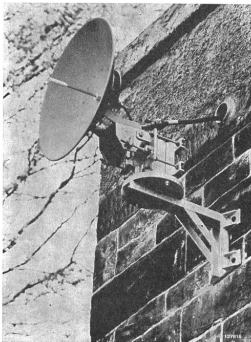
Fig. 1 Mikrowellen-Sendeempfänger mit Antenne Der parabolische Reflektor ist für eine Frequenz von rund 7 GHz ausgelegt
