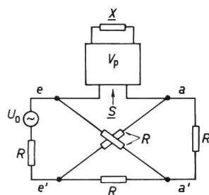
Fig. 1 Schaltung zur Phasenvervielfachung V_p beliebiges Vierpol; X Abschlussreaktanz; \underline{S} Eingangswiderstand; R Widerstand; e, e', a, a' bestimmte Punkte der Schaltung; U_0
