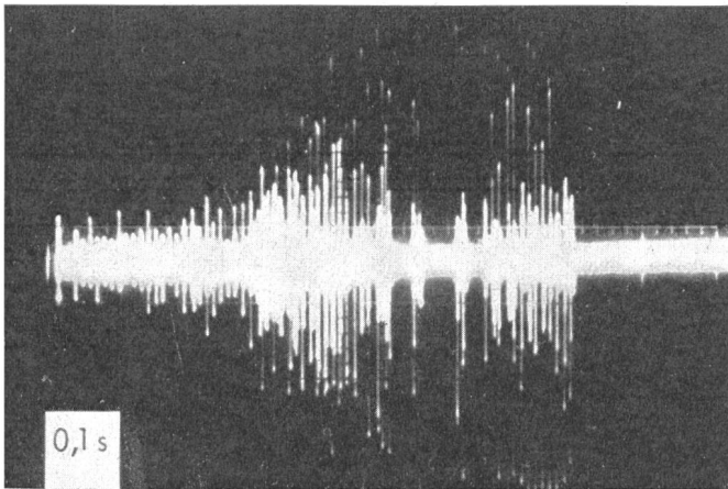
Fig. 2 Nutzsignal und Trennergeräusch gemessen am Niederfrequenzanfang eines Einseitenband-Empfängers (vor NF-Filter)
