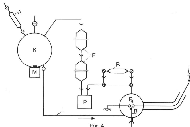
Fig. 4 Anordnung zur Messung der Durchschlagspannung «technisch reiner» Öle A Trockenrohr; K Konditionsgefäß; M Rührmotor; F Glaswatten- Filter; P Membranpumpe; P_g Prüfgefäß; P_r Ölprobengefäß für Wasserbestimmung; L Ölleitung; B Reinigungsbürste
