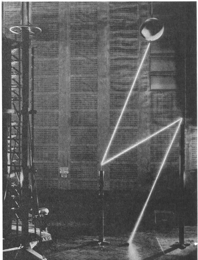
Fig. 11 Drahtverdampfen
