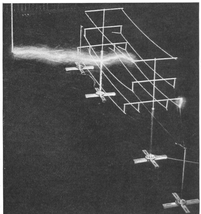
Fig. 17 Rückwärtiger Überschlag an einer Modelleitung
