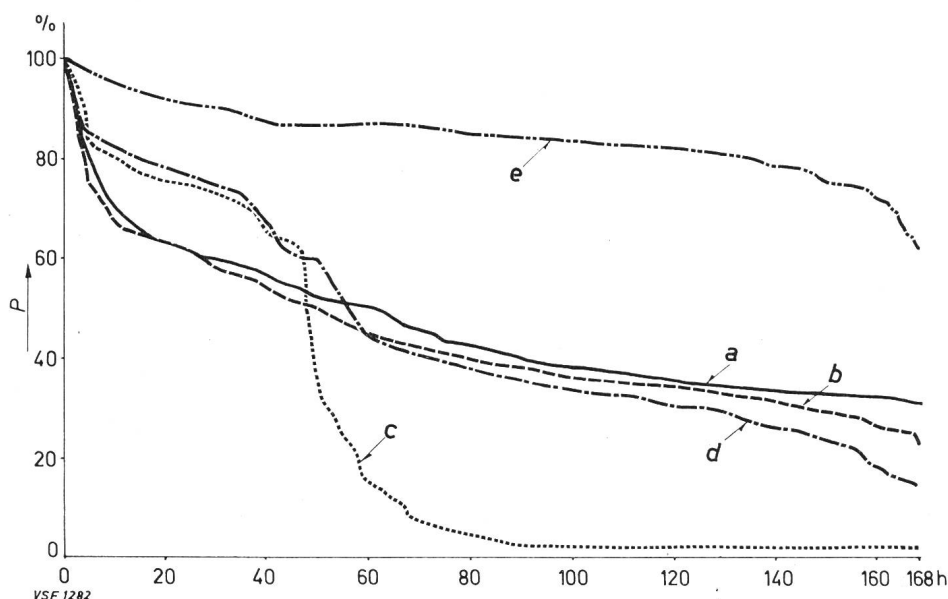
Fig. 1 Courbes monotones des charges de diverses lignes à moyenne tension (12 kV), en pourcent de la charge maximum
