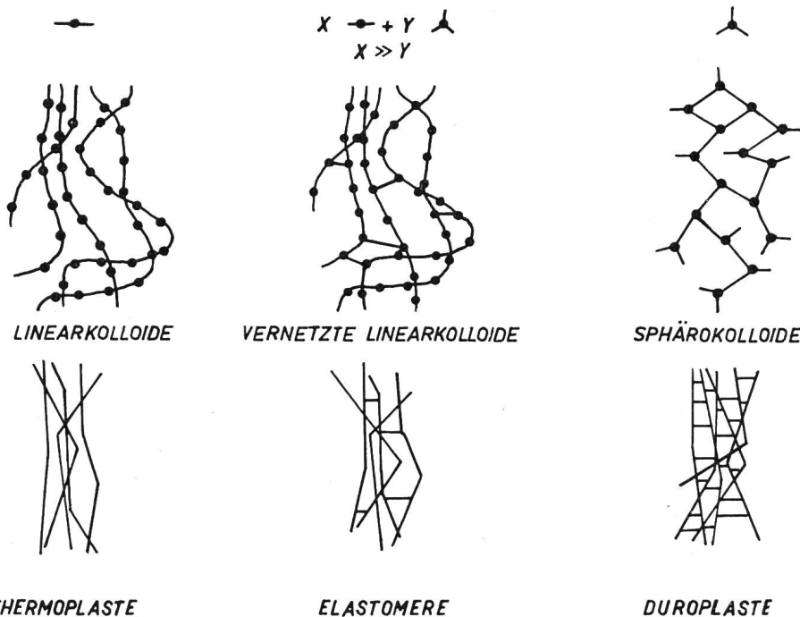
Fig. 1 Aufbau und Einteilungsprinzip makromolekularer Stoffe
