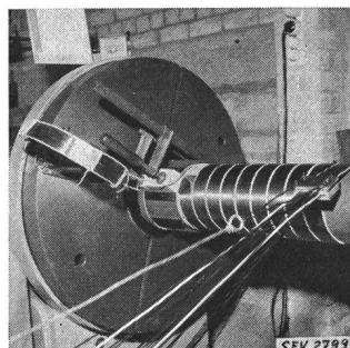
Fig. 10 Niederspannungs- Hauptwicklung 20 Cu-Drähte sind parallel geschaltet
