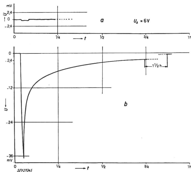
Vergleich zwischen Netzgerät in Fig. 13 und 14 und einem Bleiakкумуляtor von 6 V und 80 Ah Ladevermögen Belastung in beiden Fällen 1 A. Beim Akkumulator wurde die Belastung während einer Minute eingeschaltet a Netzgerät; b Bleiakкумуляtor U Spannung; t Zeit
