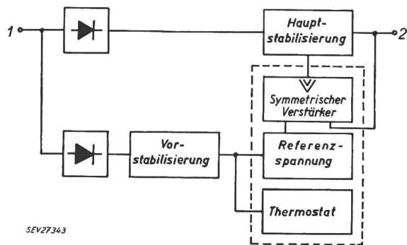
Fig. 14 Blockschema des hochstabilisierten Transistornetzgerätes der Abteilung für angewandte Physik der Universität Basel 1 Eingang; 2 Ausgang
