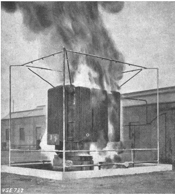
Fig. 5 Le transformateur en feu
