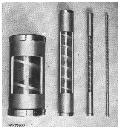
Fig. 17 Koaxialkabel
