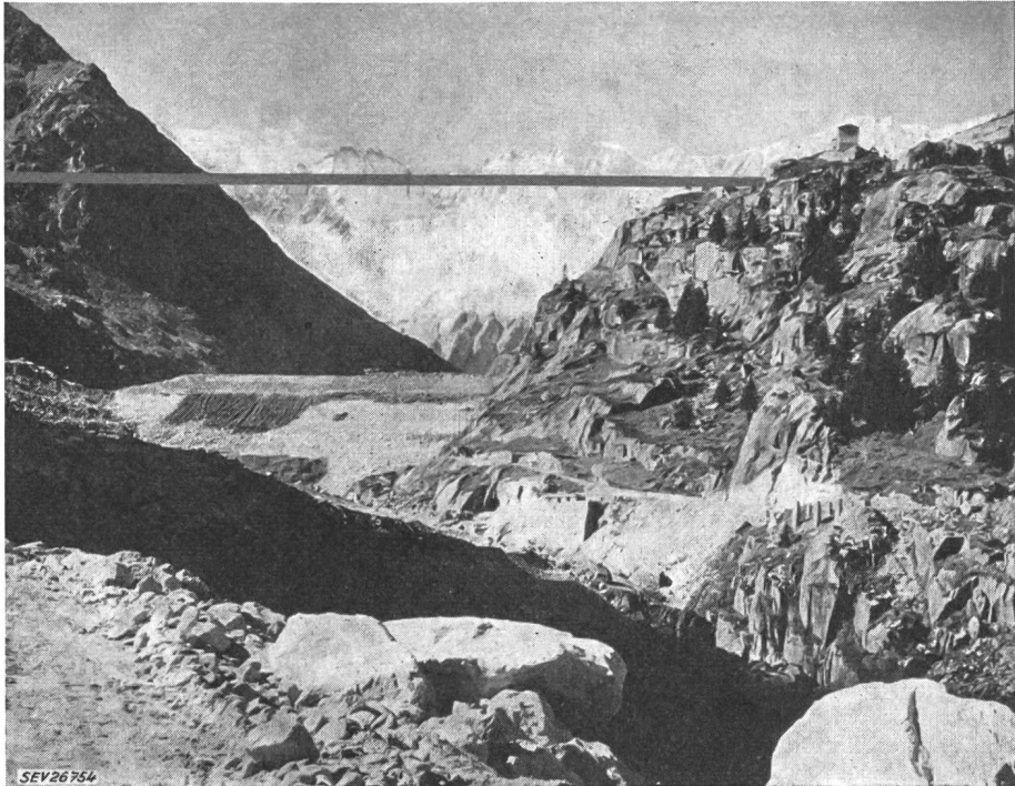
Fig. 4 Sperrstelle Göschenenalp Luftseitige Dammböschung mit angezeichneter Dammkronen Stand Oktober 1957
