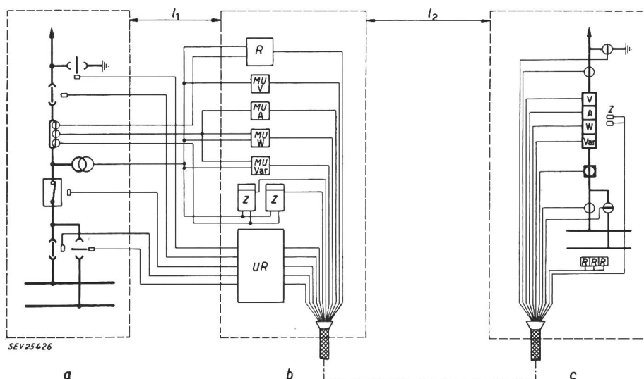
Prinzipschema der Steuerung
