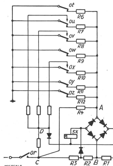
Fig. 5 Prinzip des Fehlerdetektors Bezeichnungen siehe im Text
