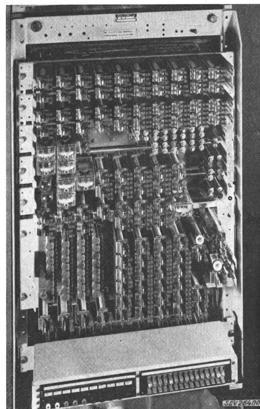
Fig. 11 TOR-Telex-Übertrager
