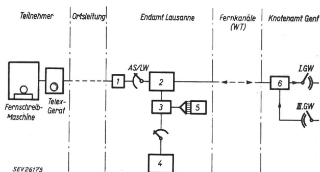
Fig. 9 Verbindungsschema Telex-Endamt Lausanne
