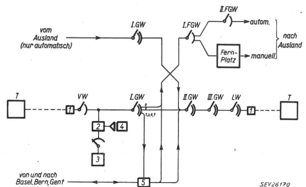
Fig. 4 Verbindungsschema der Telexzentrale Zürich 1 Umsetzer und Vorwählerschaltung; 2 Zählaktansaltung; 3 Zonen-Ausscheider; 4 zentraler Zähltakt-Geber; 5 Übertra- gung; FGW Ferngruppenwähler; VW Vorwähler; T Telex- teilnehmer
