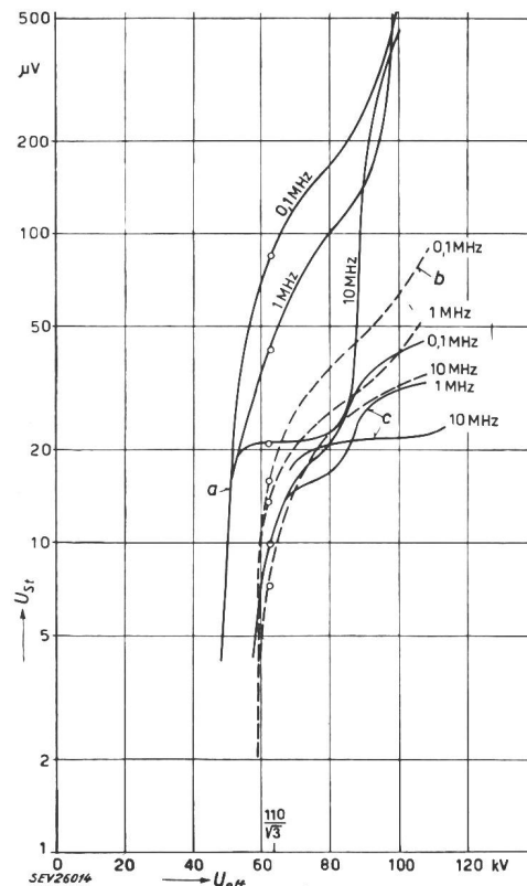
Fig. 4 Störspannung in Abhängigkeit von der Hochspannung beim Langstabisolator L 75/14
