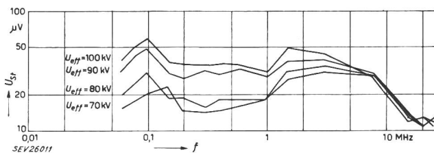
Fig. 1 Störspannung eines Langstabisolators L 75/14 ohne Schutzelektroden
