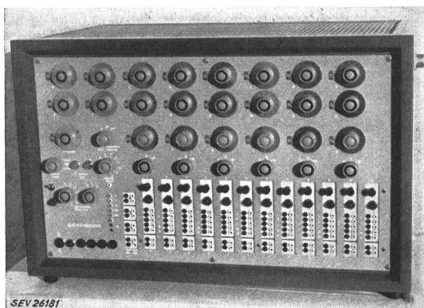
Fig. 2 Klein-Analogierechengerät
