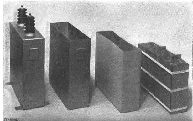
Fig. 11 Hochspannungskondensator der Condensateurs Fribourg S. A. Nennspannung 3000 V; Nennleistung 25 kVar
