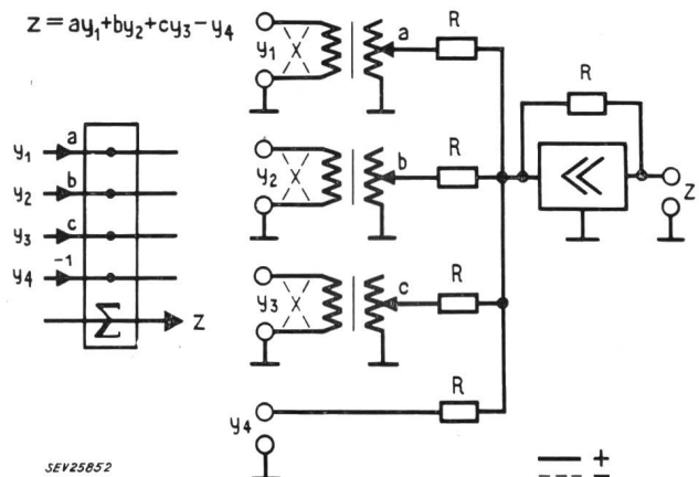
Fig. 7 Addierglied
