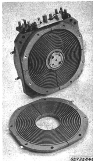
Fig. 4 Trigonometrischer Rechenkondensator
