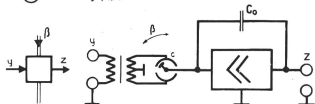
Fig. 2 Multiplikator und Funktions-Rechenkondensator
