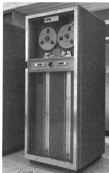
Fig. 8 Magnetbandeinheit
