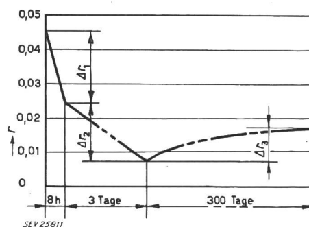
Fig. 2 Veränderung der Reaktivität r
