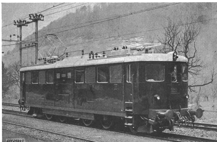
Fig. 8 Lokomotive Ae 4/6 Inbetriebnahme 1941...1945. 80 t, 4100 kW (5540 PS), v_{max} = 125 \text{ km/h}
