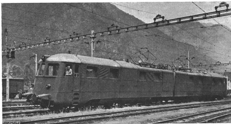
Fig. 7 Doppellokomotive Ae 8/14 Nr. 11852 Inbetriebnahme 1939. 236 t, 8800 kW (12 000 PS) (an den Motorwellen), v_{max} = 110 \text{ km/h}
