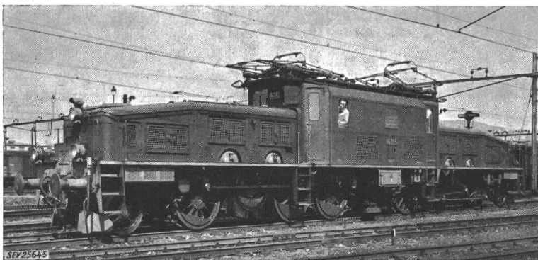
Fig. 4 Güterzuglokomotive Ce 6/8 III Baujahre 1926...1927. 131 t, 1800 kW (2460 PS) v_{max} = 65 (später 75) km/h
