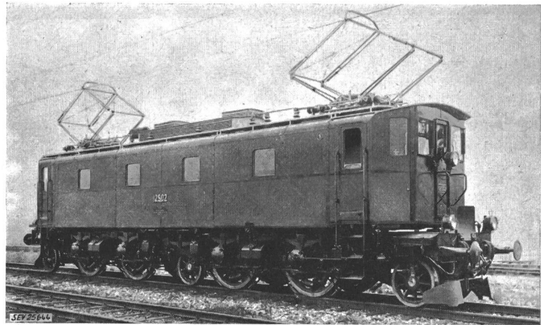
Fig. 3 Schnellzuglokomotive Be 4/7 Inbetriebnahme 1922. 110 t, 1750 kW (2400 PS), v_{max} = 75 (später 80) km/h
