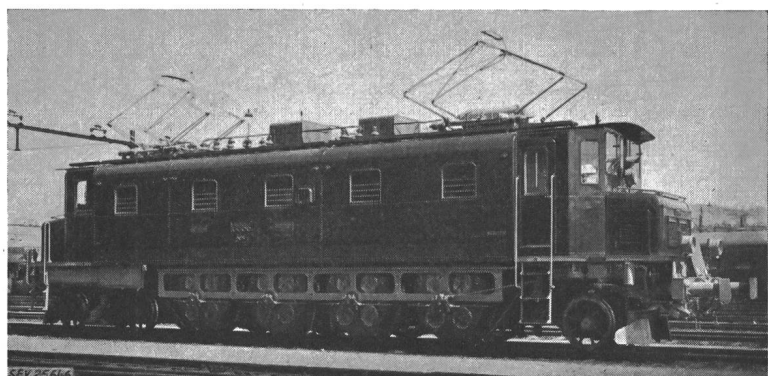
Fig. 5 Schnellzuglokomotive Ae 4/7 Baujahre 1927...1934. 123 t, 2300 kW (3120 PS), v_{max} = 100 km/h
