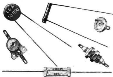
Fig. 4 Condensateurs céramique
