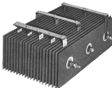
Fig. 2 «Sécheron-Selengleichrichter-Säule
