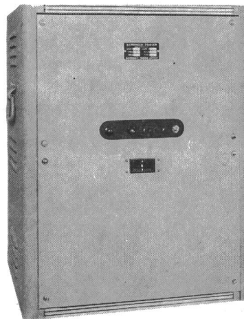
Fig. 1 Wechselspannungsregler 5000-2 S, 220/220 V, 5 kVA
