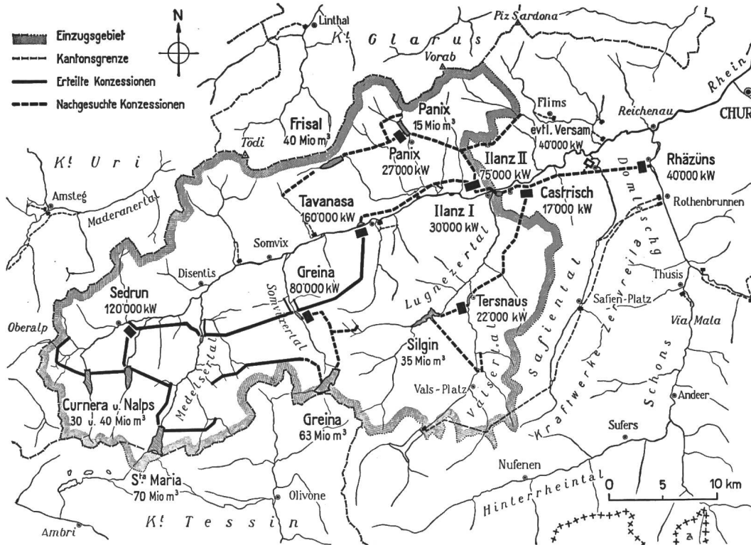
Fig. 1 Wasserkräfte des Vorderrheins, Situation
