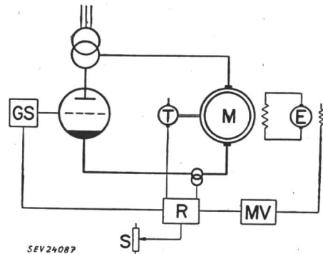
Fig. 7 Prinzipschema der modernen Steuerung eines Umkehrwalzwerkes in Eingefässhaltung mit Feldumkehr M Motor; E Rapiderreger; T Tachodynamo; R Regler; S Drehzahl-Sollwertgeber; GS magnetischer Rapid-Gittersteuersatz; MV Erreger-Magnetverstärker
