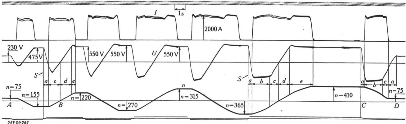
Fig. 8 Folge von Reversiervorgängen eines mutatorgesteuerten Umkehrmotors im Leerlauf I Ankerstrom; U Ankerspannung; n Drehzahl in U/min; A...B Reversieren im Ankerspannungsbereich; B...C Reversieren mit der Enddrehzahl im Feldschwächbereich; C...D Drehzahlensenkung und Wiederbeginn des Walzprogramms; S Steuerungssignal; a Feldumkehr; b Bremsen bei Feldverstärkung und konstanter Wechselrichterspannung; c Bremsen mit vollem Feld im Ankerspannungs-Regelbereich; d Anfahren im Ankerspannungs-Regelbereich; e Anfahren im Feldschwächbereich
