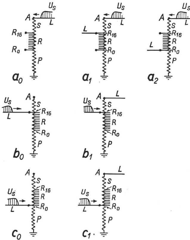
Fig. 2 Stoßschaltungen
