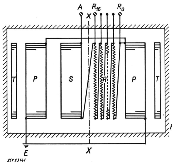
Fig. 11 Eisenfenster des Reguliersparttransformators mit Regulier- wicklung in Lagenanordnung mit 16 Stufen R_0 \dots R_{16} P Primär (Stamm-)wicklung; R Regulierwicklung; S Sekundär (Zusatz-)wicklung
