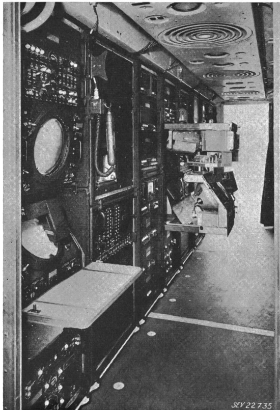
Fig. 5 Innenansicht des Radaranhängers der Fig. 4
