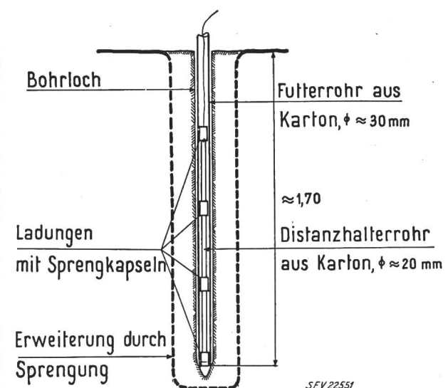
Fig. 1 Lage des Futterrohres mit Sprengladungen im Boden
