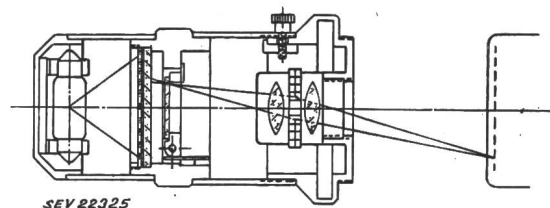
Fig. 1 Prüfprojektor mit weggklappbarem Testbild für eine Superorthikonkamera
