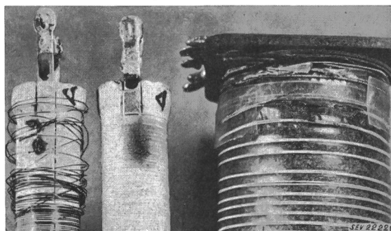
Fig. 11 Zerstörte Widerstände und Wicklungen
