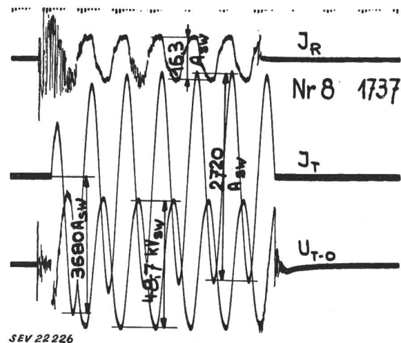
Fig. 8 Oszillogramm von Versuch 8. Erdschlussstrom und Phasenspannung von Phase T sowie Strom Phase R der Leitung Airolo-Mörel
