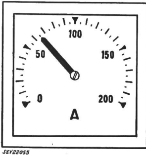
Fig. 5 Quadratisches Schalttafelinstrument mit zentraler Ringskala von 250°
