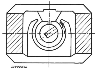
Fig. 6 Drehpulinstrument mit Hakenpol zur Erzielung eines Skalenwinkels von 250°
