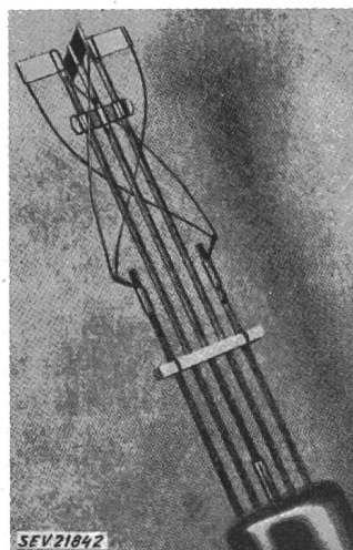
Fig. 2 Neue Kathodenform
