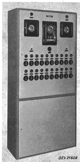
Fig. 8 Kommandoschrank, ausgebaut für 20 Doppelbefehle
