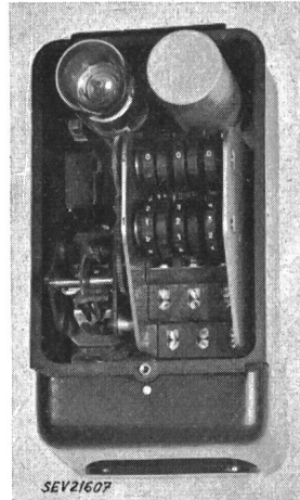
Fig. 7 Netzkommandoempfänger für 3 Doppelbefehle (System Ghielmetti)
