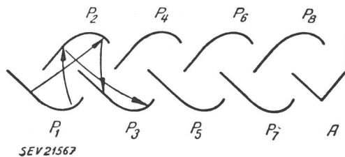
Fig. 7 Schematischer Aufbau des Vervielfachers in Fig. 6 A Anode; P_1 \dots P_8 Dynoden
