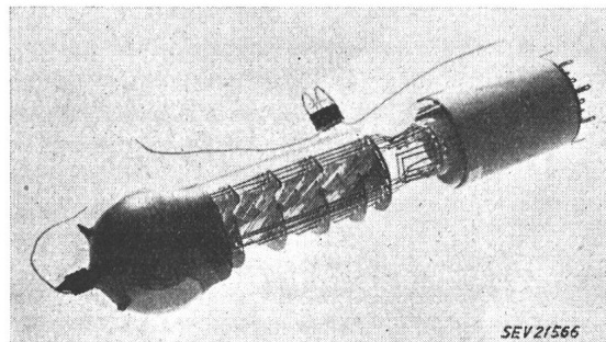
Fig. 6 17stufiger Elektronenvervielfacher mit Li-Sb-Kathode
