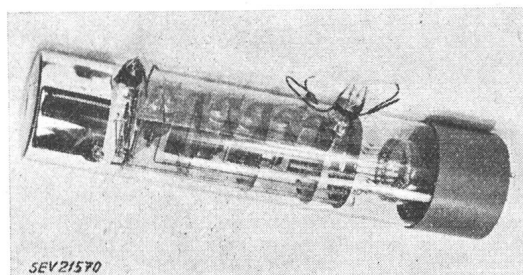
Fig. 10 12stufiger Vervielfacher
