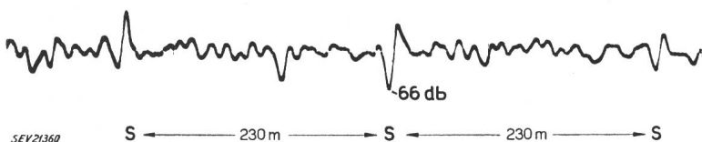
Fig. 20 Rückflussspannungen auf einem Koaxialkabel 2,64/9,52 mm, herrührend von einem \sin^2 -förmigen Sendeimpuls mit einer Halbwertzeit von 0,05 \mu\text{s} Abszisse: Entfernung vom Kabelanfang Ordinate: Rückflussschwankung A_r = 20 \cdot \log \frac{2 Z_0}{\Delta Z}
