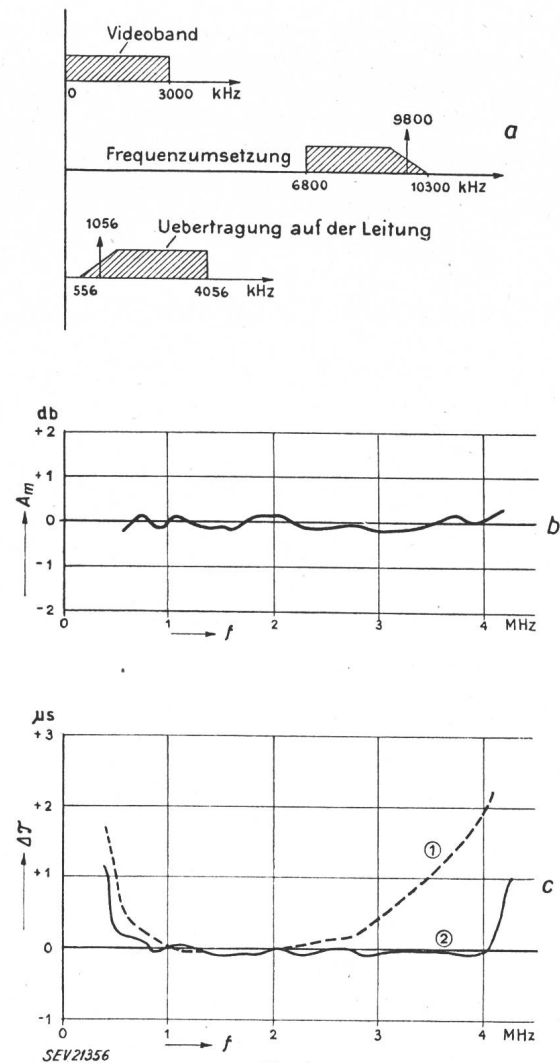
Fig. 16 Koaxialkabelanlage Birmingham-Manchester nach [15] a Modulationsschema für die Fernsehübertragung; b Betriebsdämpfung A_m in Funktion der Frequenz; c Verzerrung der Gruppenlaufzeit \Delta\tau in Funktion der Frequenz; 1 ohne Laufzeitentzerrung; 2 mit Laufzeitentzerrung
