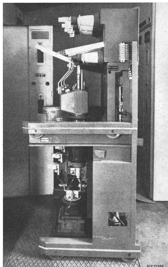
Fig. 6 Schaltwagen
