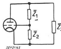
Fig. 6 Ersatzschema der Spannungsteiler- oder Dreipunktschaltung
