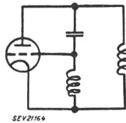
Fig. 5 Induktive Dreipunktschaltung oder Hartley-Oszillator
