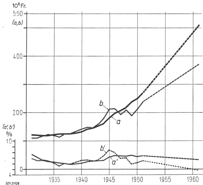
Fig. 6 Total der ertragsunabhängigen und ertragsabhängigen Ausgaben a ertragsunabhängige Ausgaben in 10^6 Fr.; a' in % der Erstellungskosten; b ertragsabhängige Ausgaben in 10^6 Fr.; b' in % der Erstellungskosten
