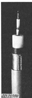
Fig. 16 Câble à isolation polythène pour la transmission de la haute tension continue (100 kV) (avec conducteur supplémentaire au centre)
