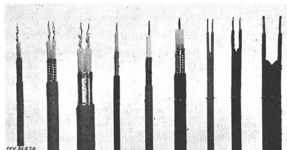
Fig. 5 Câbles d'antennes
