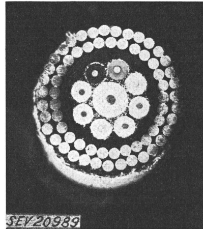
Fig. 17 Câble spécial à isolation polythène pour la station d'étude de la foudre au San Salvatore ( 1 \times 7 \text{ mm}^2 + 8 \times 2,5 \text{ mm}^2 ) Armure en cuivre mi-dur de 546 \text{ mm}^2 de section
