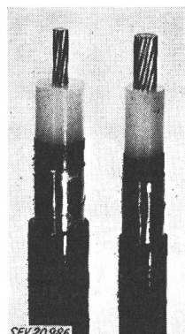
a) b) Fig. 13 Câble à haute tension à isolation polythène a 25 mm 2 — 20/11,5 kV b 50 mm 2 — 10/6 kV
