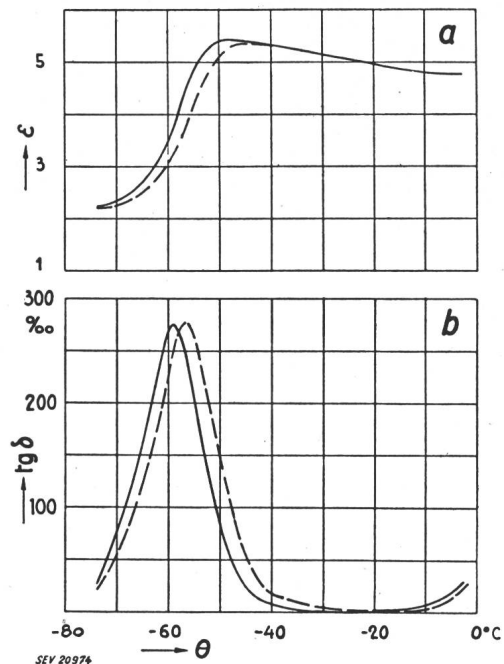
Fig. 2 Constante diélectrique ( \epsilon ) et angle de pertes ( \text{tg } \delta ) à basse température du plastifiant Di-2-éthyl-hexyl-phthalate ——— f = 800 \text{ Hz} ; - - - - f = 1600 \text{ Hz}
