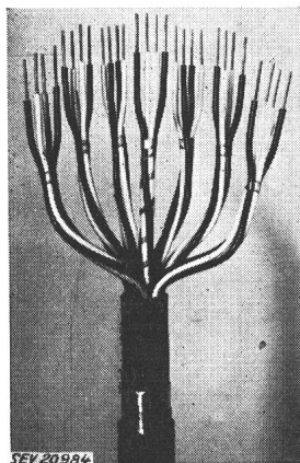
Fig. 11 Câble téléphonique à isolation polythène pour la transmission d'ondes porteuses ( 7 \times 4 \times 1,3 mm)
