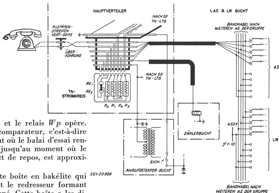
Fig. 9 Schéma de la réglette de raccordement du distributeur principal montrant le système de fiches sur lesquelles se glissent les jacks de ligne des abonnés. On reconnait l'absence totale de jacks de rupture dans ce dis- positif
