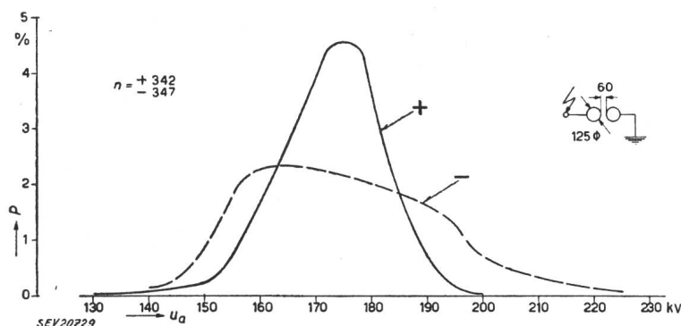
Fig. 29 Courbe de fréquence des tensions d'amorçage de l'éclateur à sphères de 125 mm de diamètre (nettoyées), à axe horizontal, représenté sur la fig. 5
