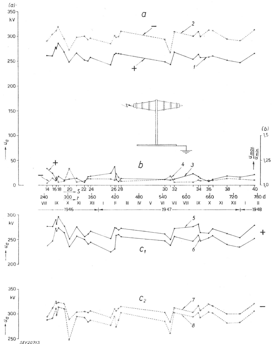
Fig. 13 Tension de contournement de la traversée représentée sur la fig. 3 a, b et c, comme pour la fig. 11
