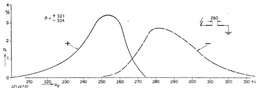
Fig. 30 Courbe de fréquence des tensions d'amorçage de l'éclateur à tiges représenté sur la fig. 6
