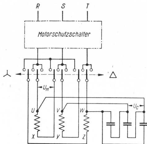
Fig. 4 Kondensator in \Upsilon - \Delta -Anlauf Nicht zu empfehlende Schaltung
