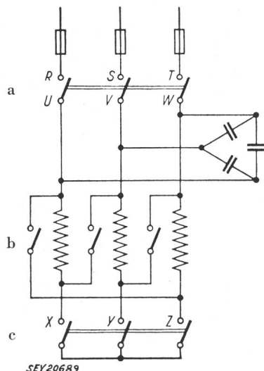
Fig. 5 Blindstrom- kompensation in \Upsilon - und \Delta -Schaltung
