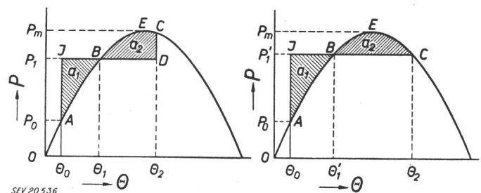
Fig. 6 Dynamische Stabilität bei Belastungsschwankung von P_0 \dots P_1 Erklärungen siehe im Text
