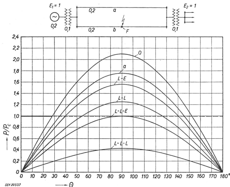
Fig. 7 Dynamische Stabilität verschiedener Betriebsfälle
