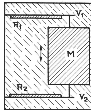
Fig. 7 Aufnehmer mit variablen Widerständen für Messung von Beschleunigungen
